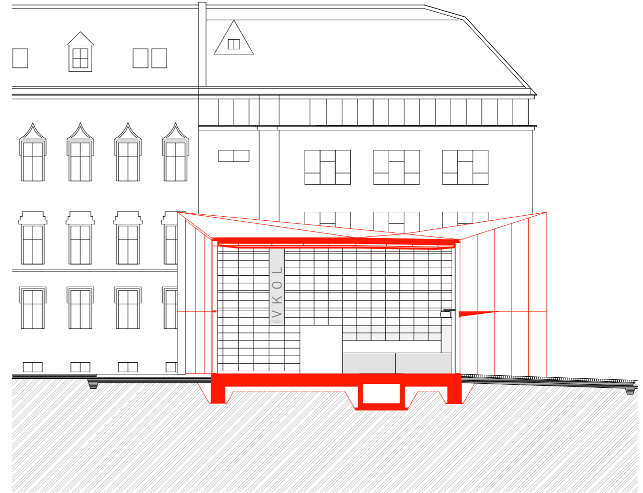
řez b-b'
